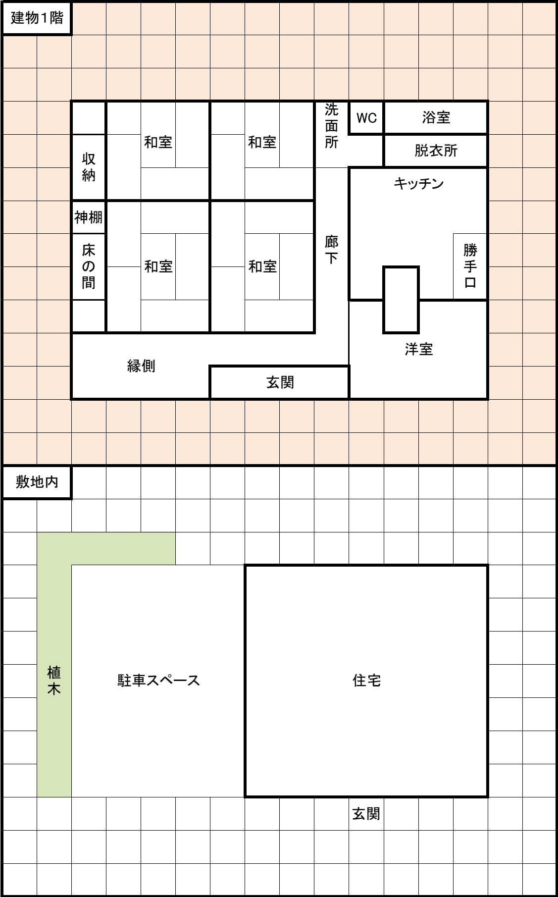
間取り図
