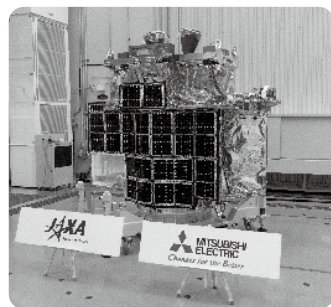
小型月着陸実証機「SLIM」の機体
